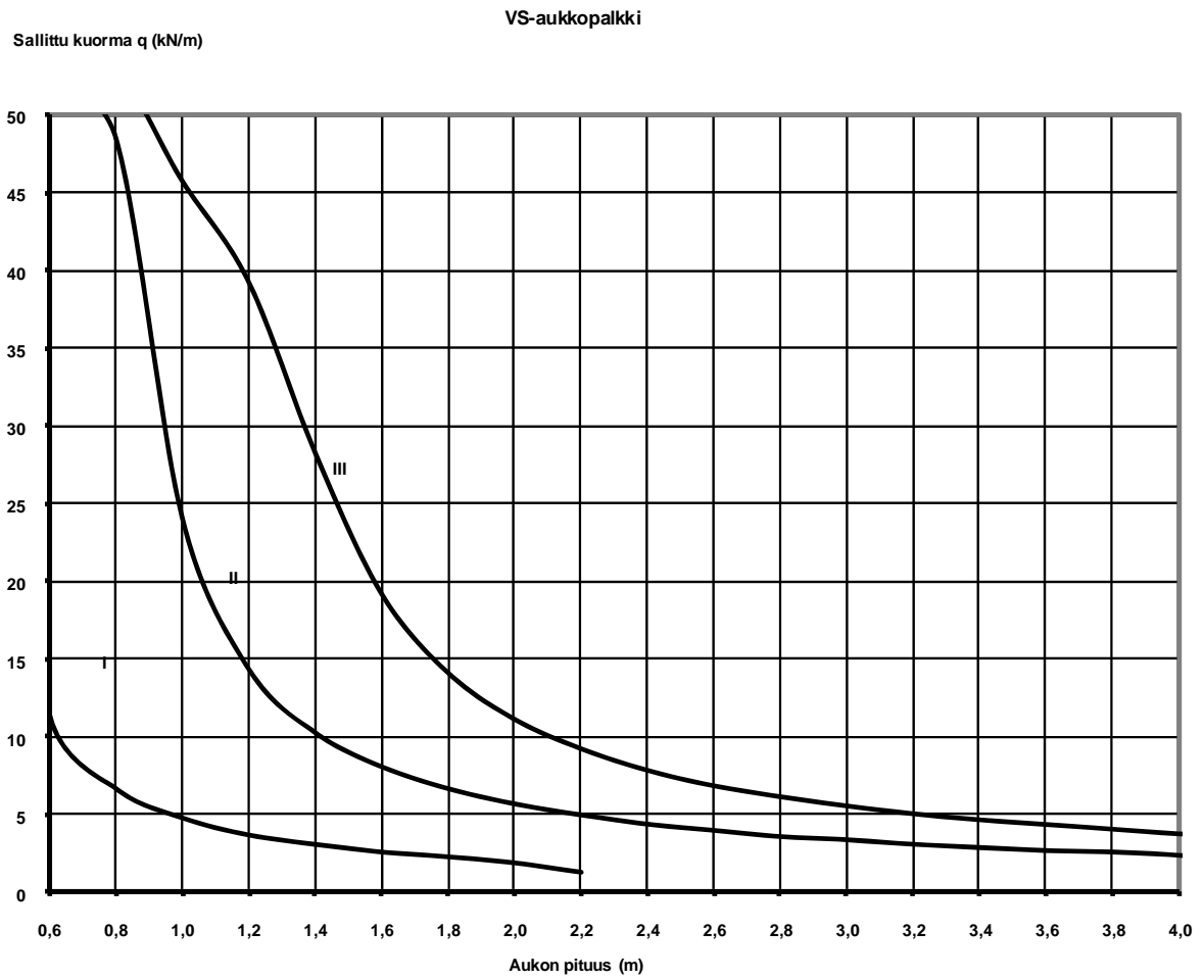
Kuva 3. Valetun palkin sallitut kuormat.
