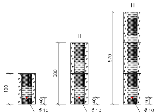
Kuva 2. Eri palkkikorkeudet
